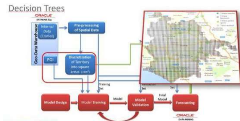
Obrázek 30: Rozhodovací stromy
